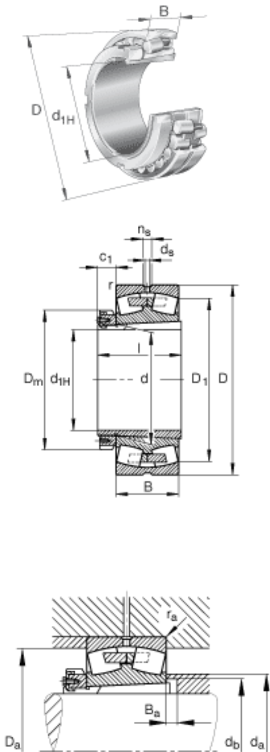
FAG 230/530-B-K-MB + H30/530图片
