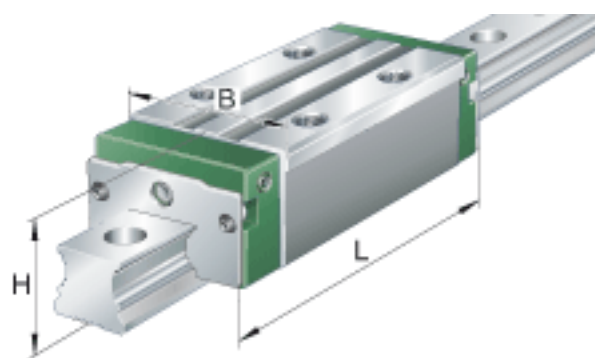
INA KWVE20-B-S图片
