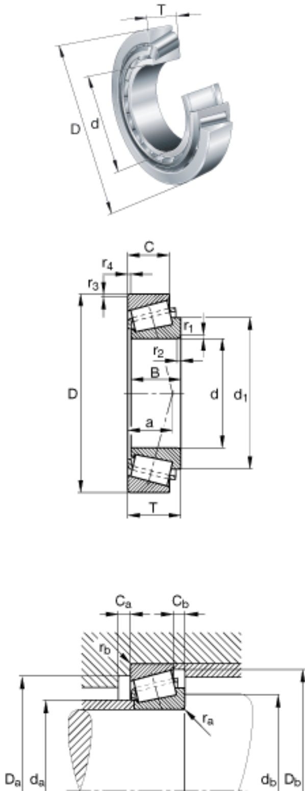
FAG 32314-A图片
