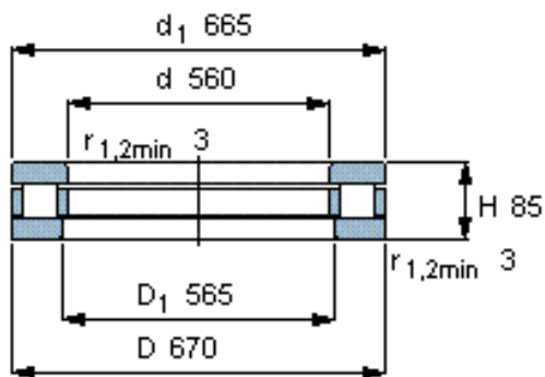
完整轴承
